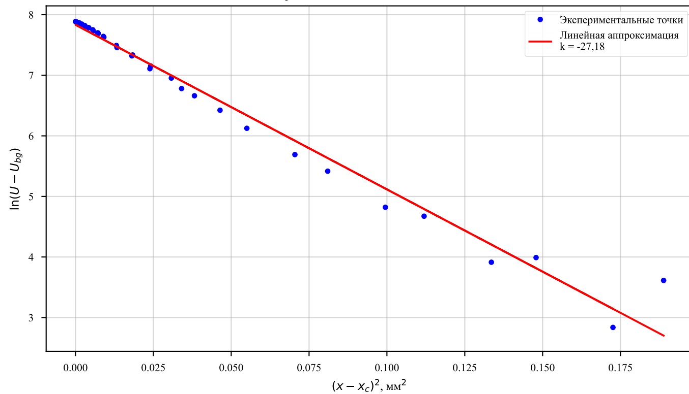
Линеаризация зависимости для z = 79,7 см
