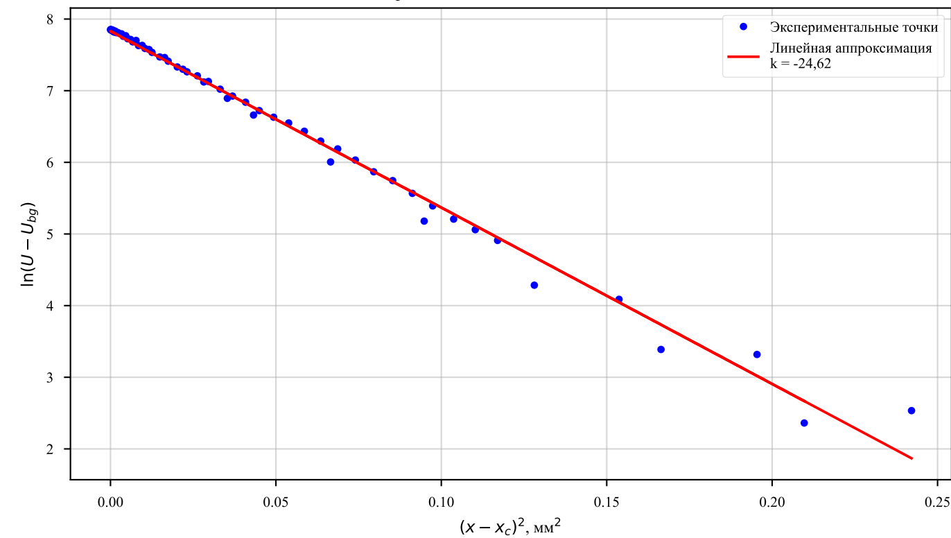
Линеаризация зависимости для z = 49,2 см
